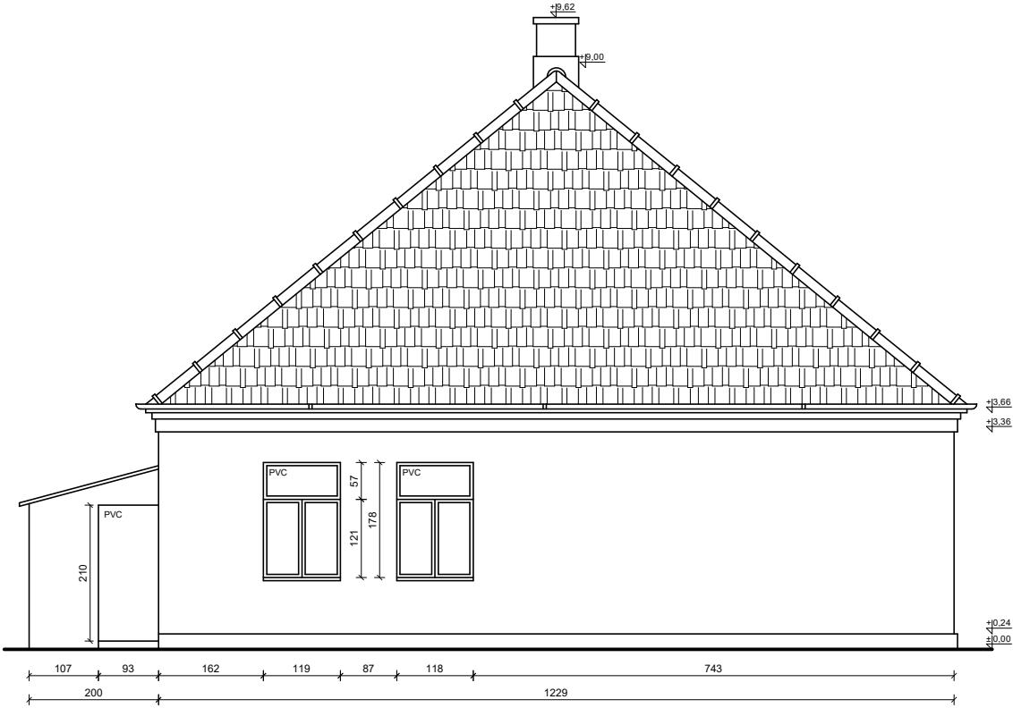
ELEWACJA POŁUDNIOWA - kolorystyka
